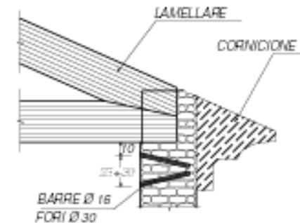
SEZIONE B-B
