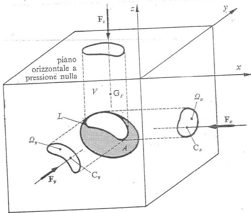
Fig. 6.6. - Decomposizione e calcolo delle spinte idrostatiche contro una superficie gobba.
