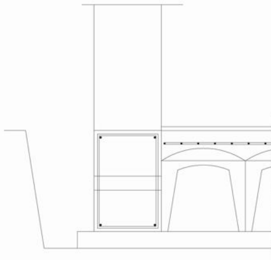
Sezione (Tipologia 2)
