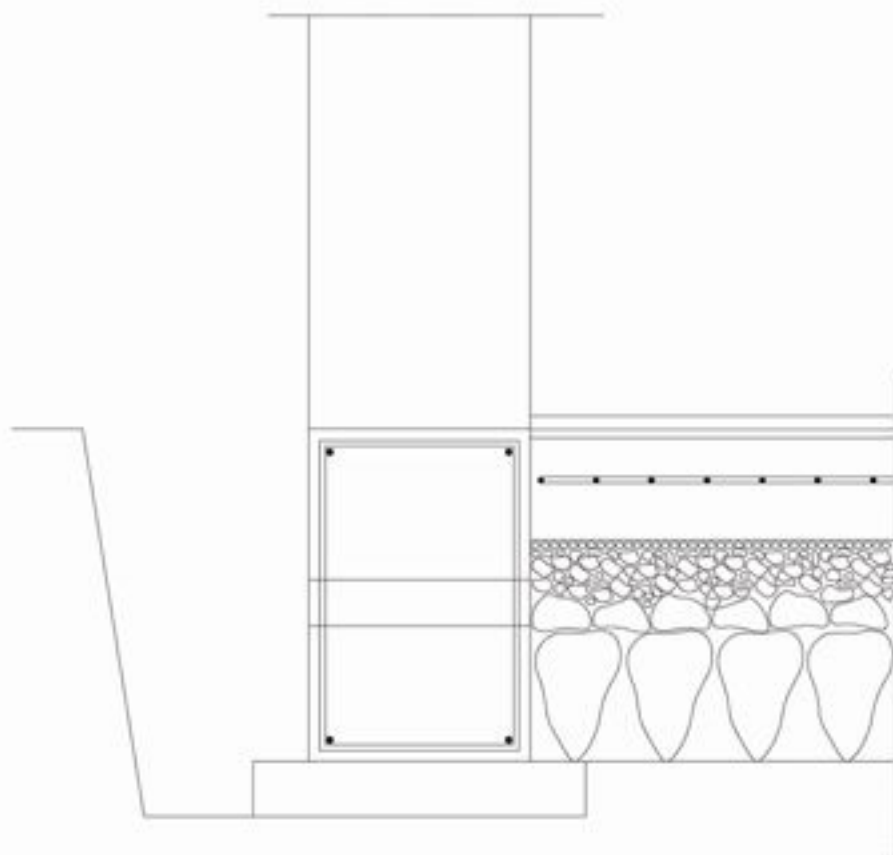
Sezione (Tipologia 1)
